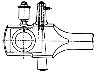
Č. 1711. Hlava ojnicní.
